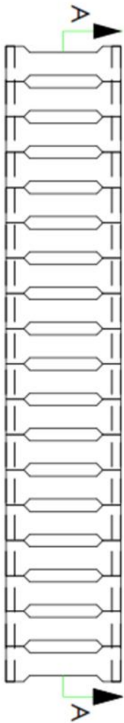
PLANTA DE CUNETA CON QUIEBRAPATAS
