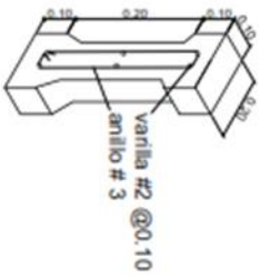
ISOMETRICO
