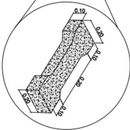
ISOMETRICO DE CUNETA CON QUIEBRAPATAS
