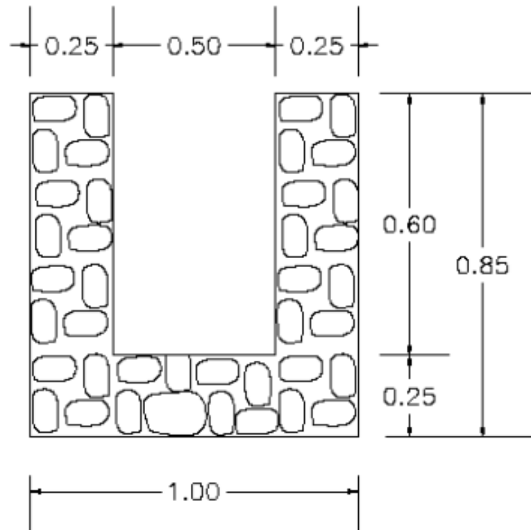
DETALLE CUNETA MAMPOSTERIA
