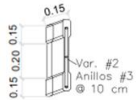
Vista isométrica
