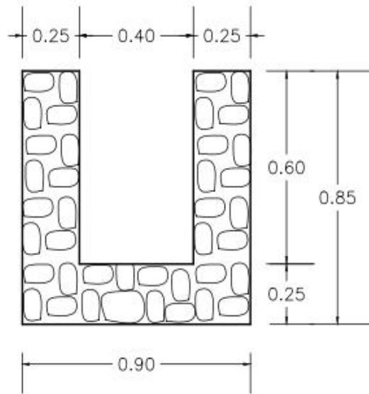
DETALLE CUNETAS MAMPOSTERIA
