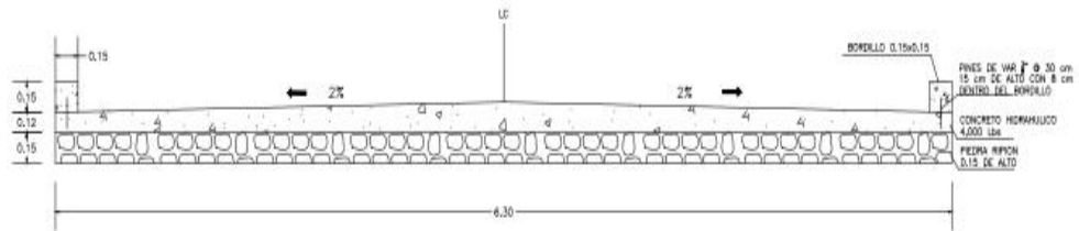
DETALLE DE WHITE TOPPING sin escala
