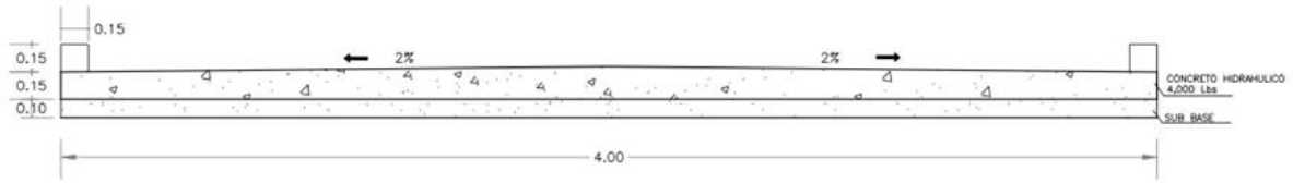
CALLE DE CONCRETO HIDRAULICO sin escala
