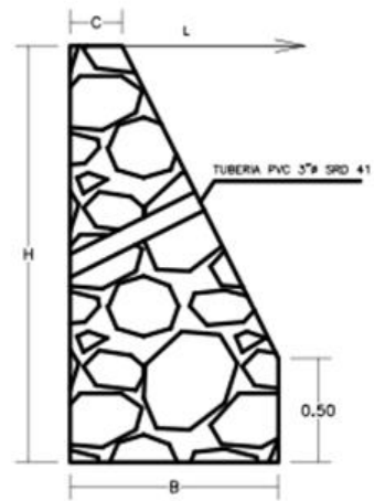
DETALLE DE MURO DE CONTENCIÓN
