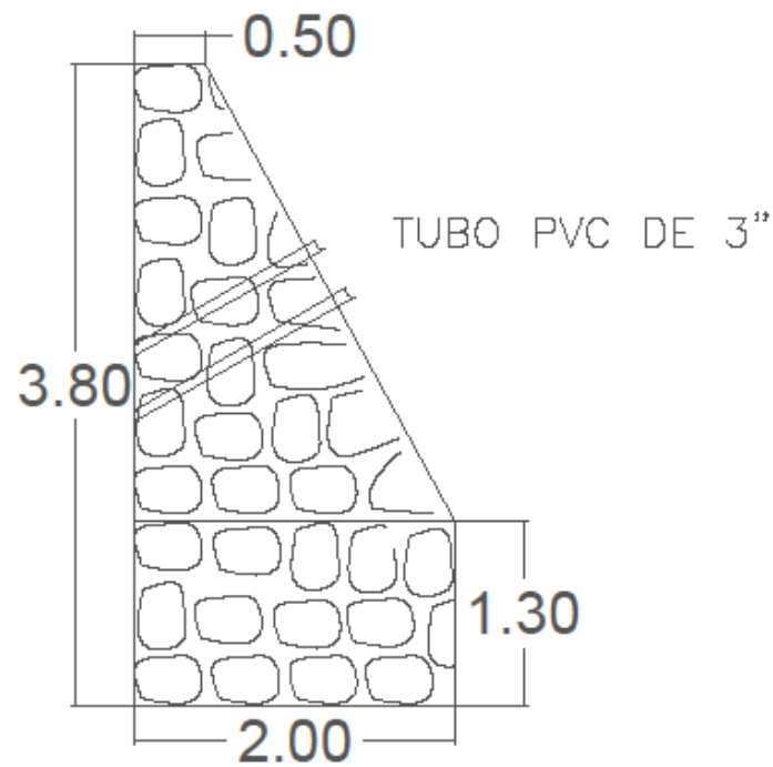
DETALLE DE MURO DE MAMPOSTERIA
