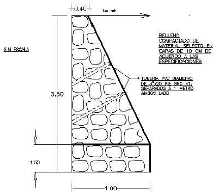
DETALLE DE MURO DE MAMPOSTERIA
