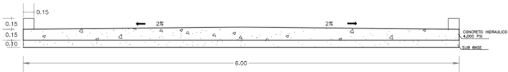
CALLE DE CONCRETO HIDRAULICO sin escale
