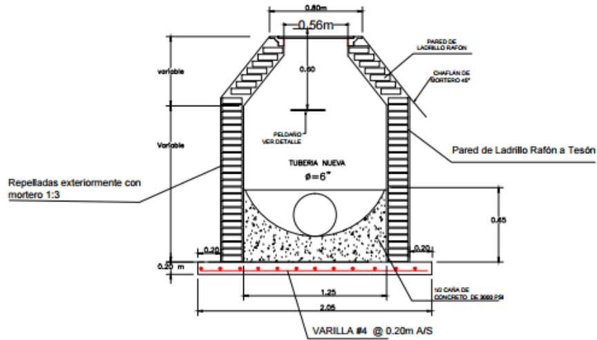
ARMADO EN BASE PARA POZOS
