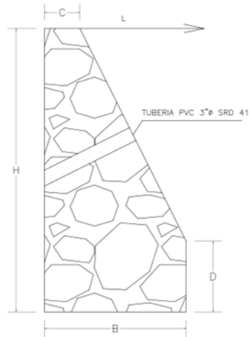
DETALLE DE MURO DE CONTENCIÓN
