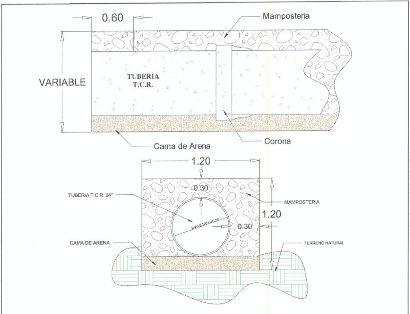
Detalle de tubería T.C.R. de 24"
