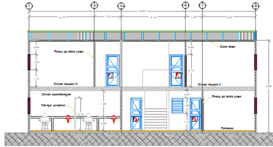
SECCION B-B Escala 1:200
