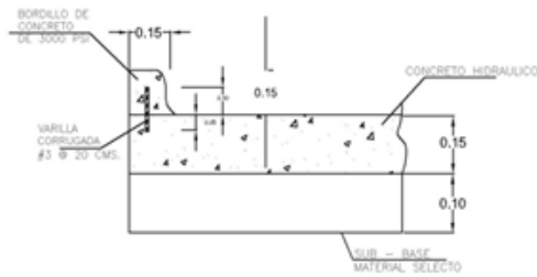
DETALLE BORDILLO DE 15 CM X 15 CM
