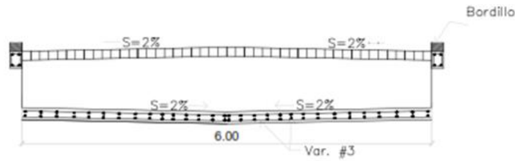
CORTE A-A
