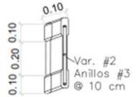
Vista isométrica
