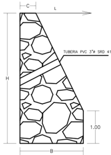
DETALLE DE MURO DE CONTENCIÓN
