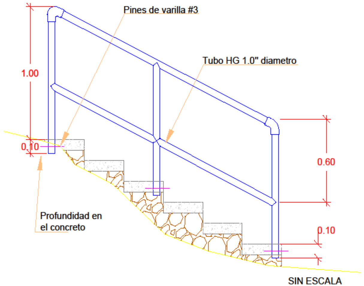
DETALLE DE PASAMANOS-GRADAS
