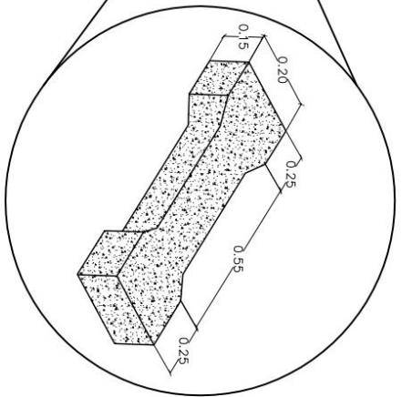
ISOMETRICO DE CUNETETA CON QUIEBRAPATAS
