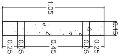
ELEVACION LATERAL
