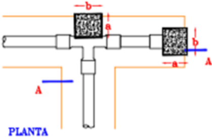
PLANTA
