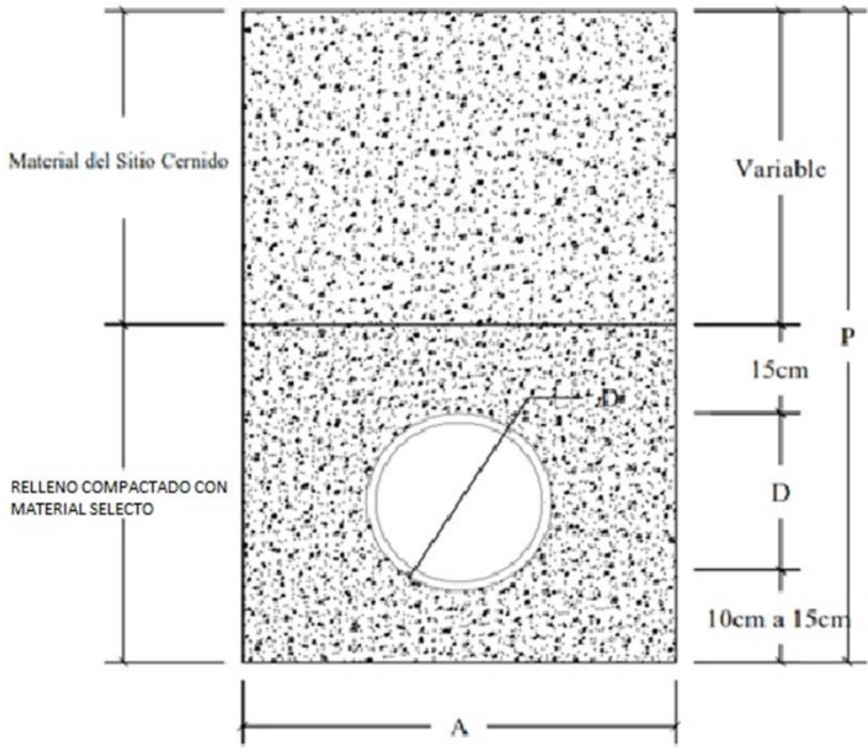
Dimensiones de los Zanjos Según el Diámetro de las Tuberías
