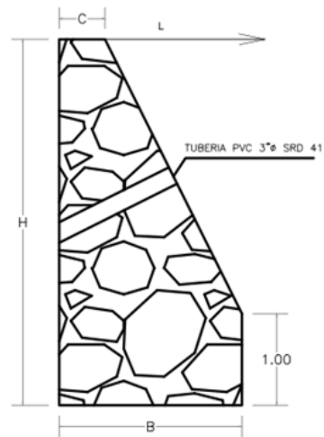
DETALLE DE MURO DE CONTENCIÓN
