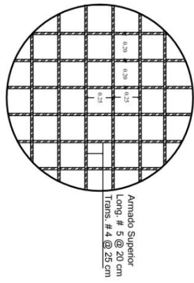
DETALLE DE LOSA, ARMADO SUPERIOR
