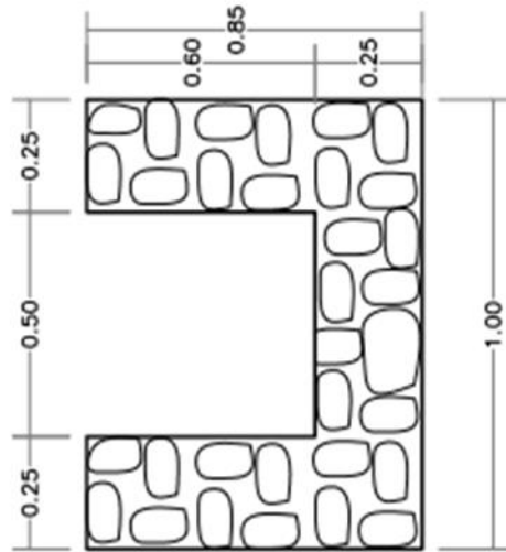
DETALLE CUNETETA
