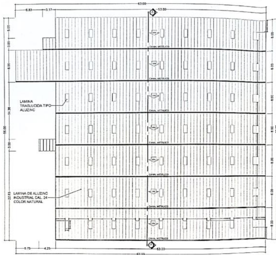
PLANTA DE TECHOS MERCADO SAN ISIDRO | ESC. 1/400
