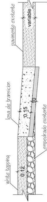
DETALLE DE LOSA DE TRANSICION
