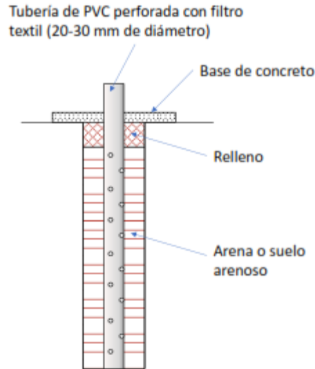
Figura 2: Ejemplo de la Especificación para tubería PVC perforada
