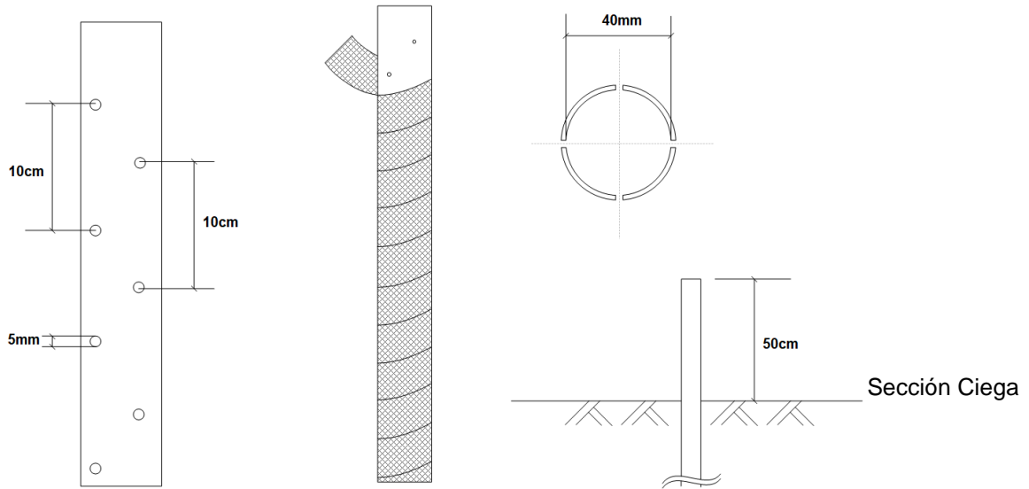
Figura: Ejemplo de la Especificación para tubería PVC perforada
