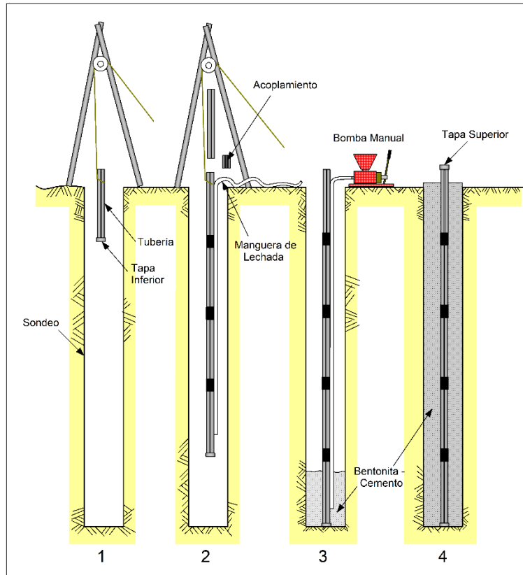
Figura: Ejemplo del Procedimiento para Instalación de Tubería Inclinométrica
