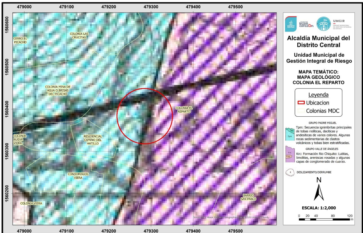
Ilustración 2. Mapa Geológico de la Colonia El Reparto donde se observa el contraste de los Grupo Padre Miguel y Valle de Ángeles.
