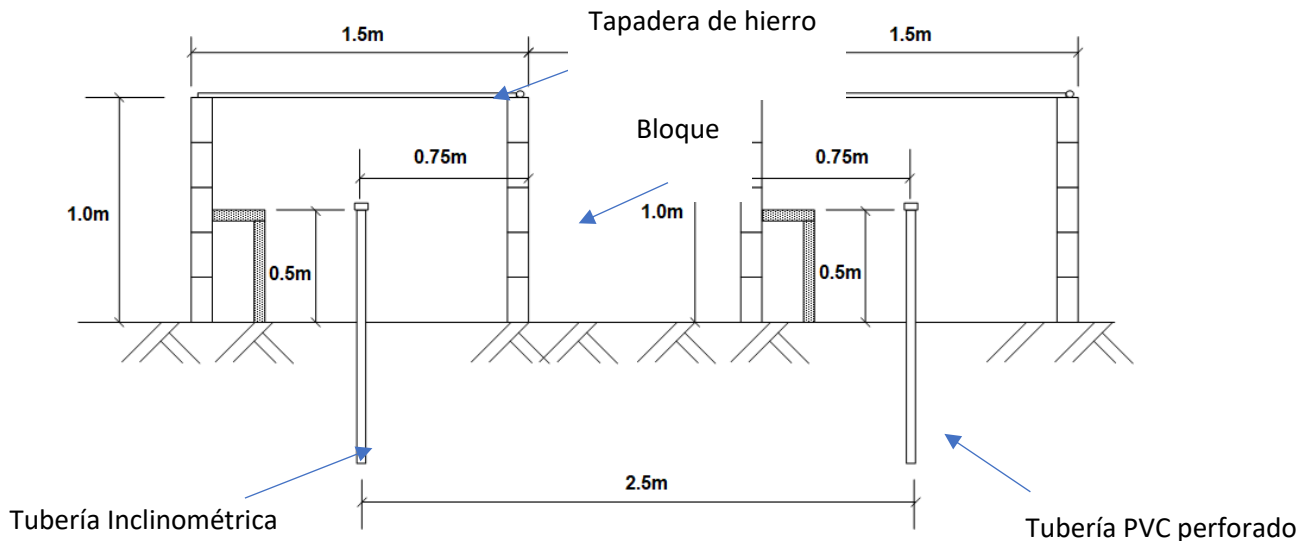
Figura: Ejemplo de las cajas de protección.
