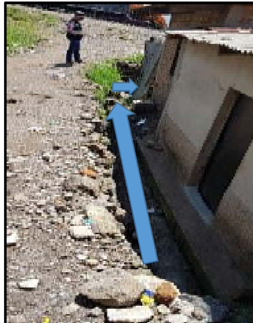
Ilustración 2. Tramo J - K; Ubicación de Cuneta a Construir (Sección 0.30m x 0.30m).
