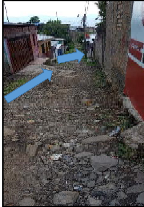
Ilustración 11. Tramo H - I; Ubicación de Cuneta a Construir (Sección 0.30m x 0.30m).
