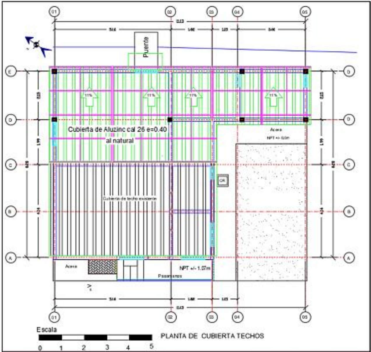
Planta de cubierta de techos a Instalar
