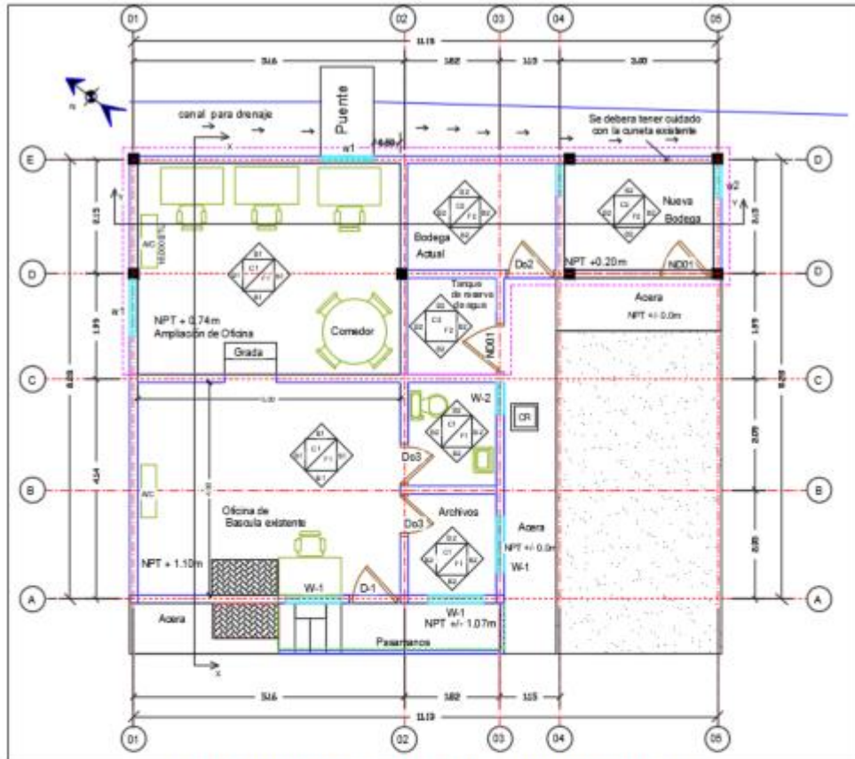
Planta constructiva de ampliación de las oficinas y bodega
