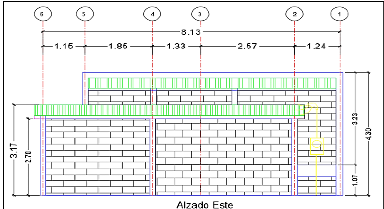
Estado actual de la fachada Posterior
