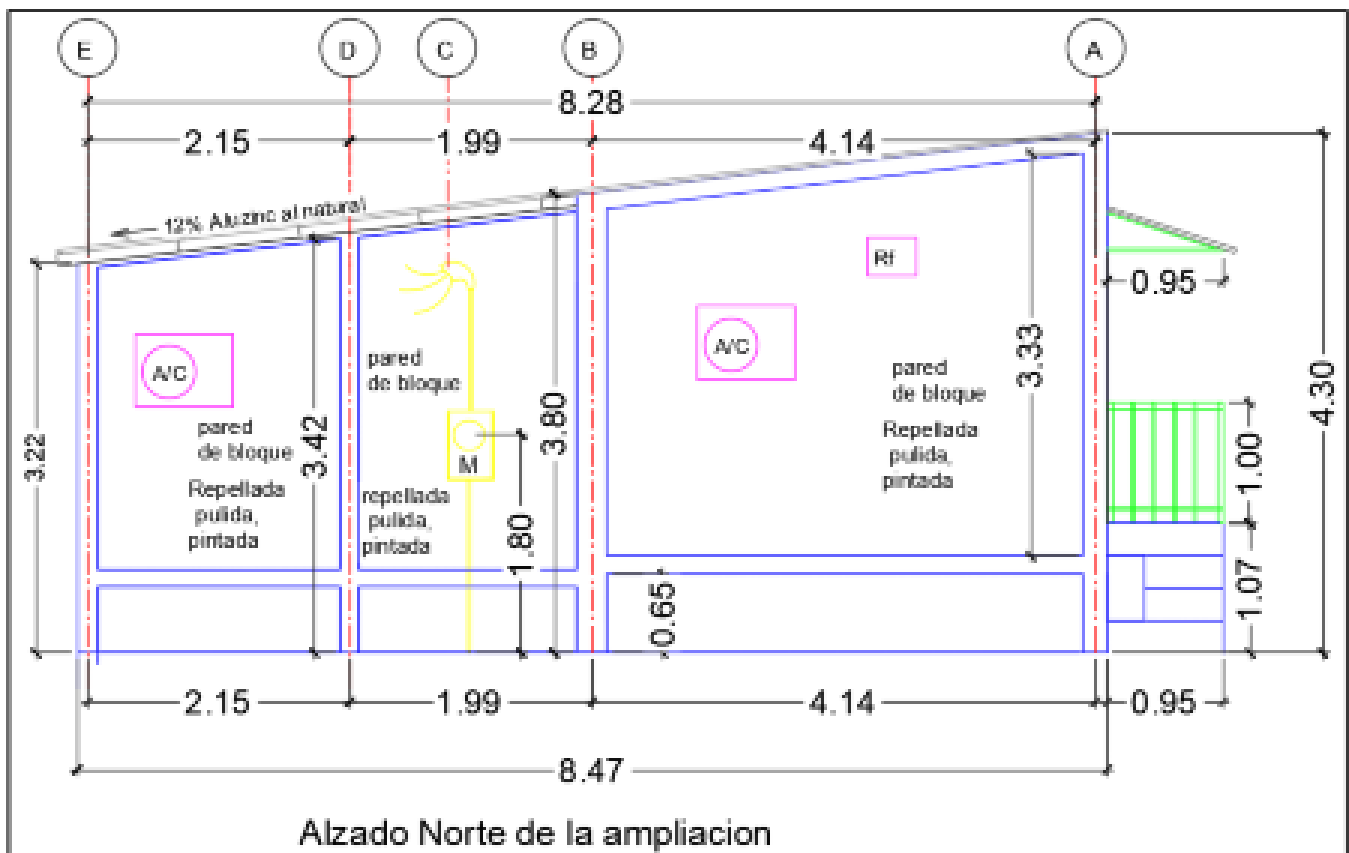
Alzado Norte Estado actual de la fachada lateral derecha
