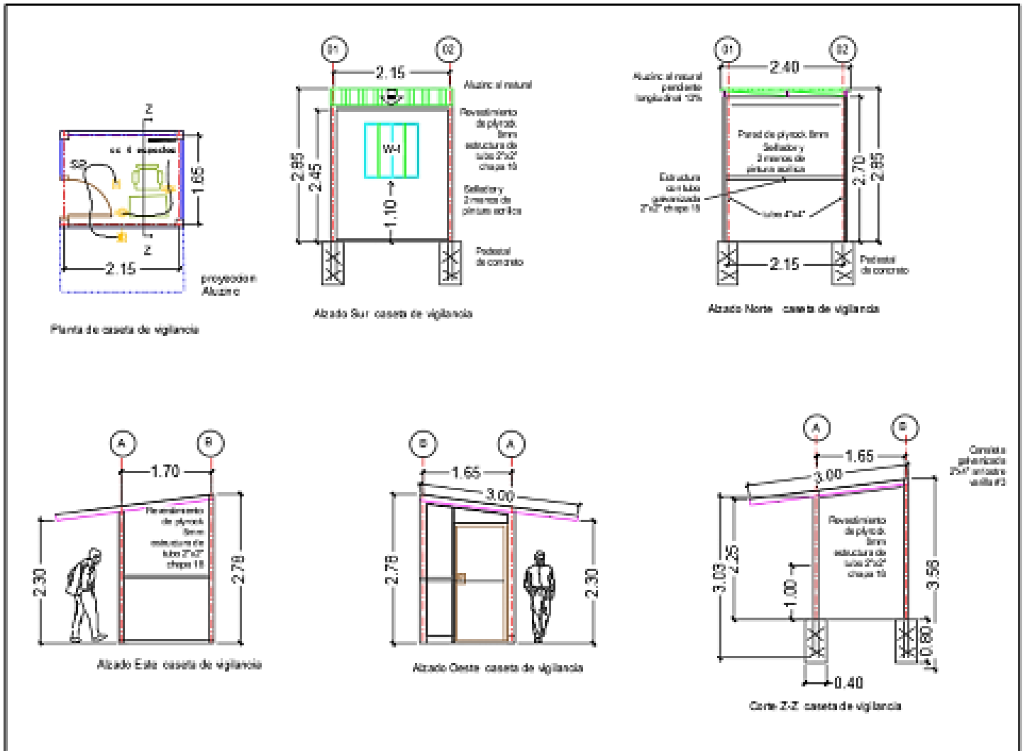
DETALLE CONSTRUCTIVO DE CASETA DE VIGILANCIA
