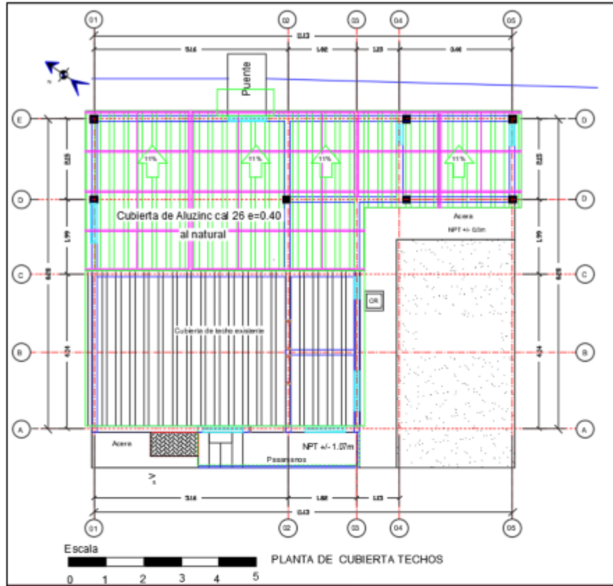
Planta de cubierta de techos a Instalar
