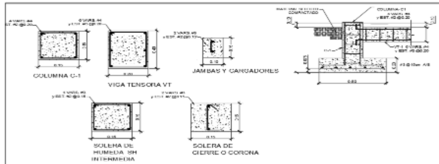
PLANTA DE CIMENTACION Y DETALLES ESTRUCTURALES
