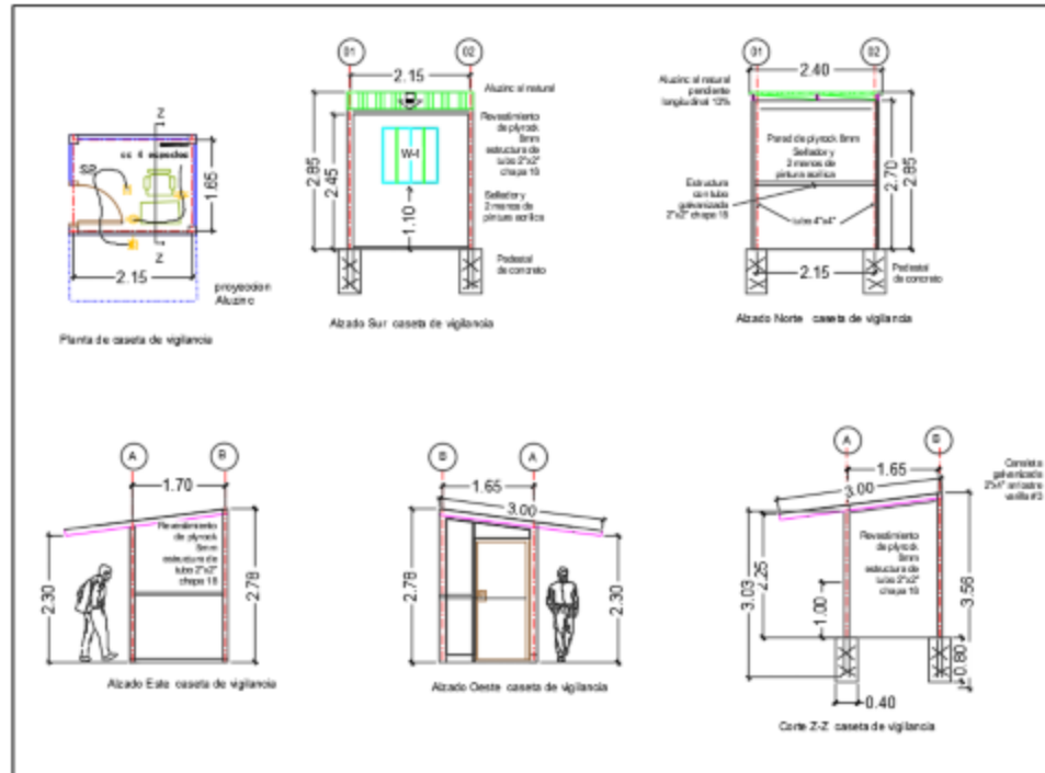
DETALLE CONSTRUCTIVO DE CASETA DE VIGILANCIA
