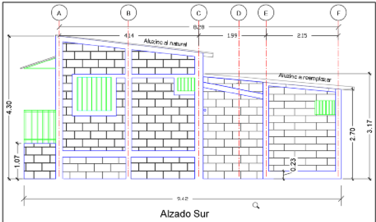
Estado actual de la fachada lateral izquierda
