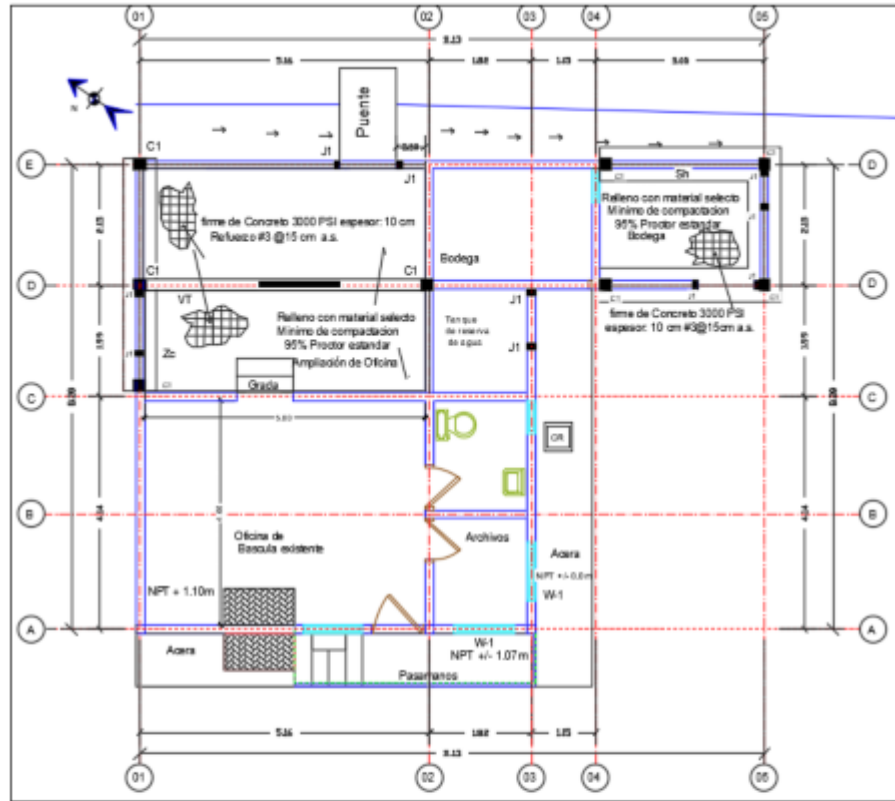
PLANTA DE CIMENTACION Y DETALLES ESTRUCTURALES
