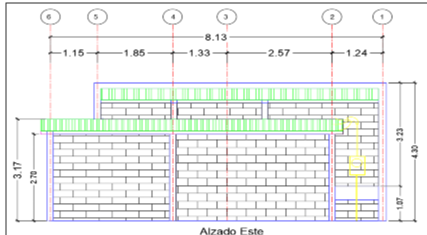
Estado actual de la fachada Posterior
