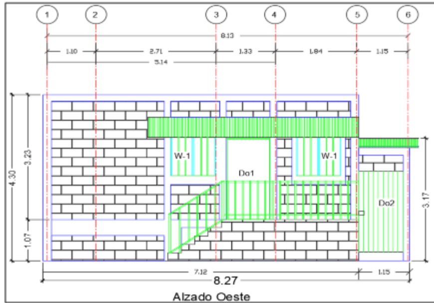
Estado actual de la fachada frontal
