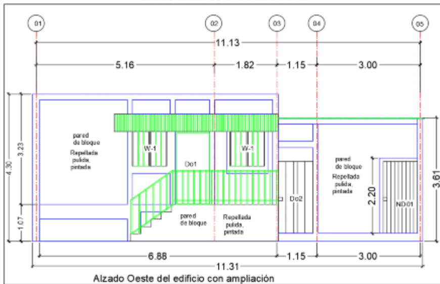
Alzado Oeste del edificio con ampliación
