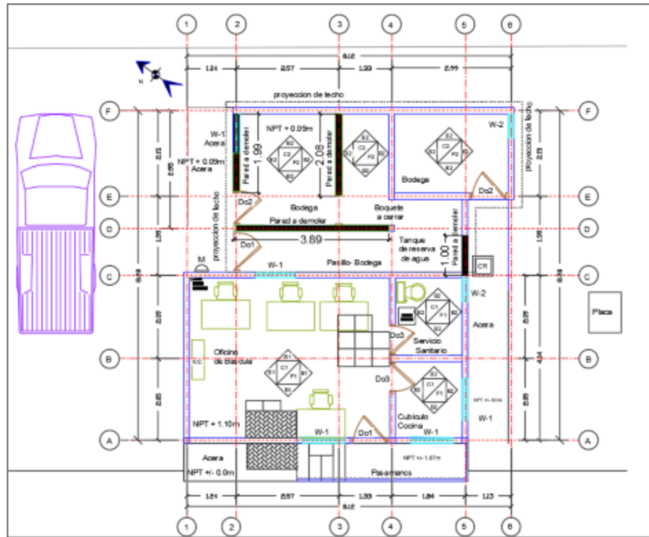
Planta constructiva de la situación actual de las oficinas y bodega
