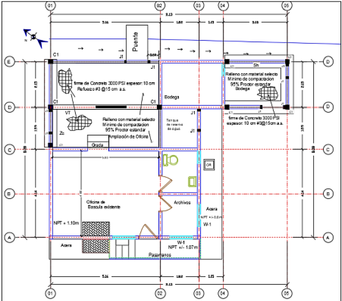
PLANTA DE CIMENTACION Y DETALLES ESTRUCTURALES
