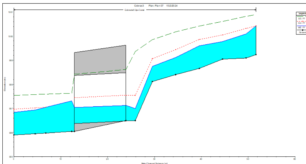
Perfil Hidráulico de Caja 2 Propuesta
