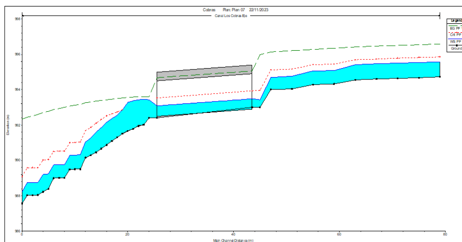
Perfil Hidráulico de Caja 2 Propuesta
