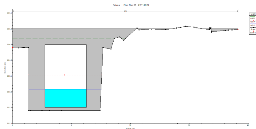
Sección Transversal Caja 1 Propuesta
