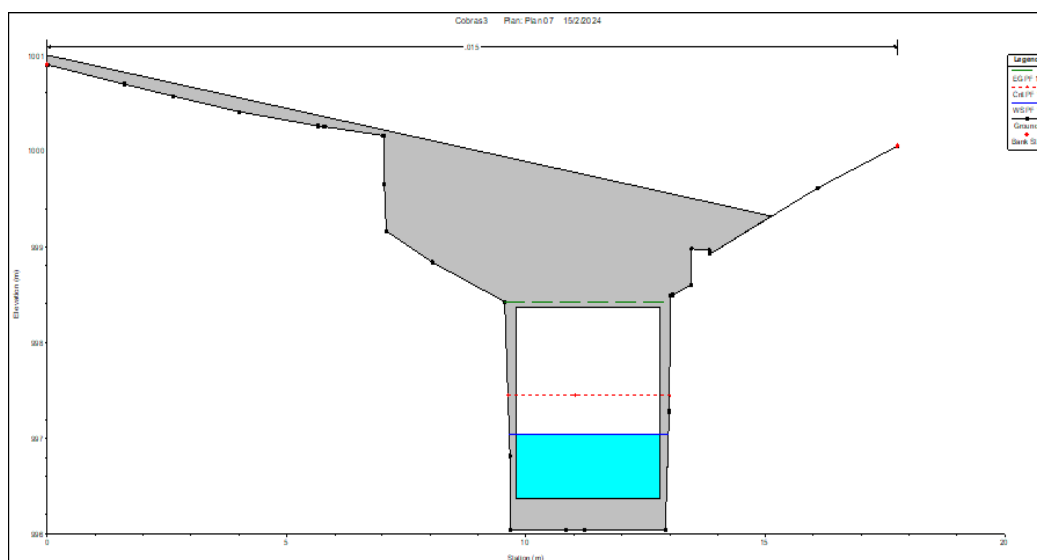
Sección Transversal Caja 2 Propuesta
