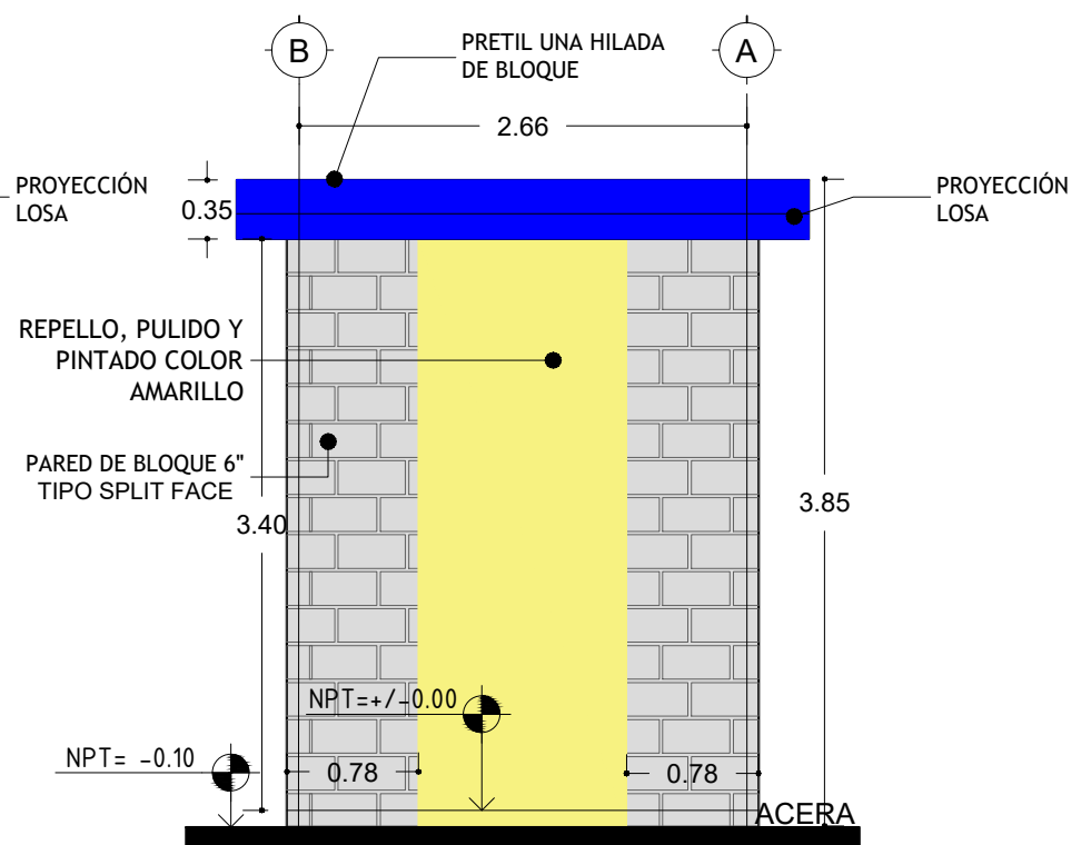
FACHADA LATERAL IZQUIERDA CUARTO ELECTRICO
