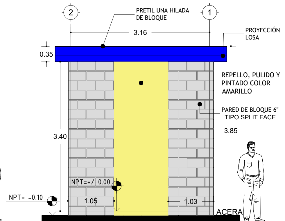
FACHADA POSTERIOR CUARTO ELECTRICO
