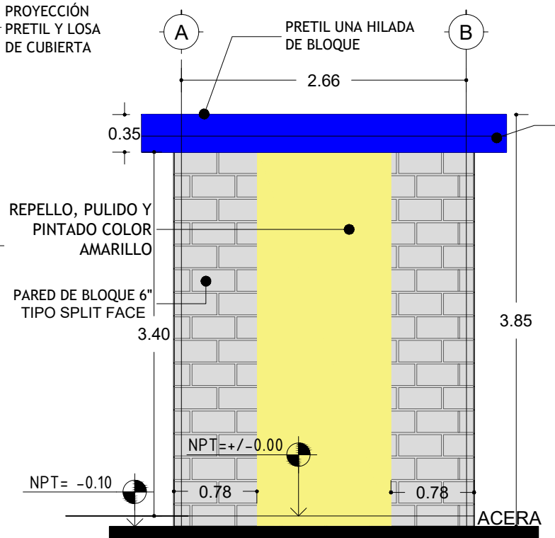
FACHADA LATERAL DERECHA CUARTO ELECTRICO
