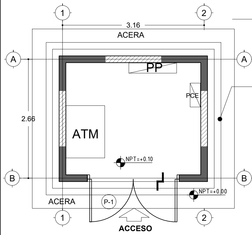
PLANTA ARQUITECTÓNICA CUARTO ELECTRICO
