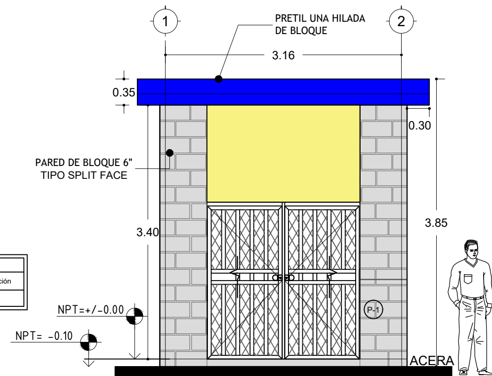
FACHADA FRONTAL CUARTO ELECTRICO
