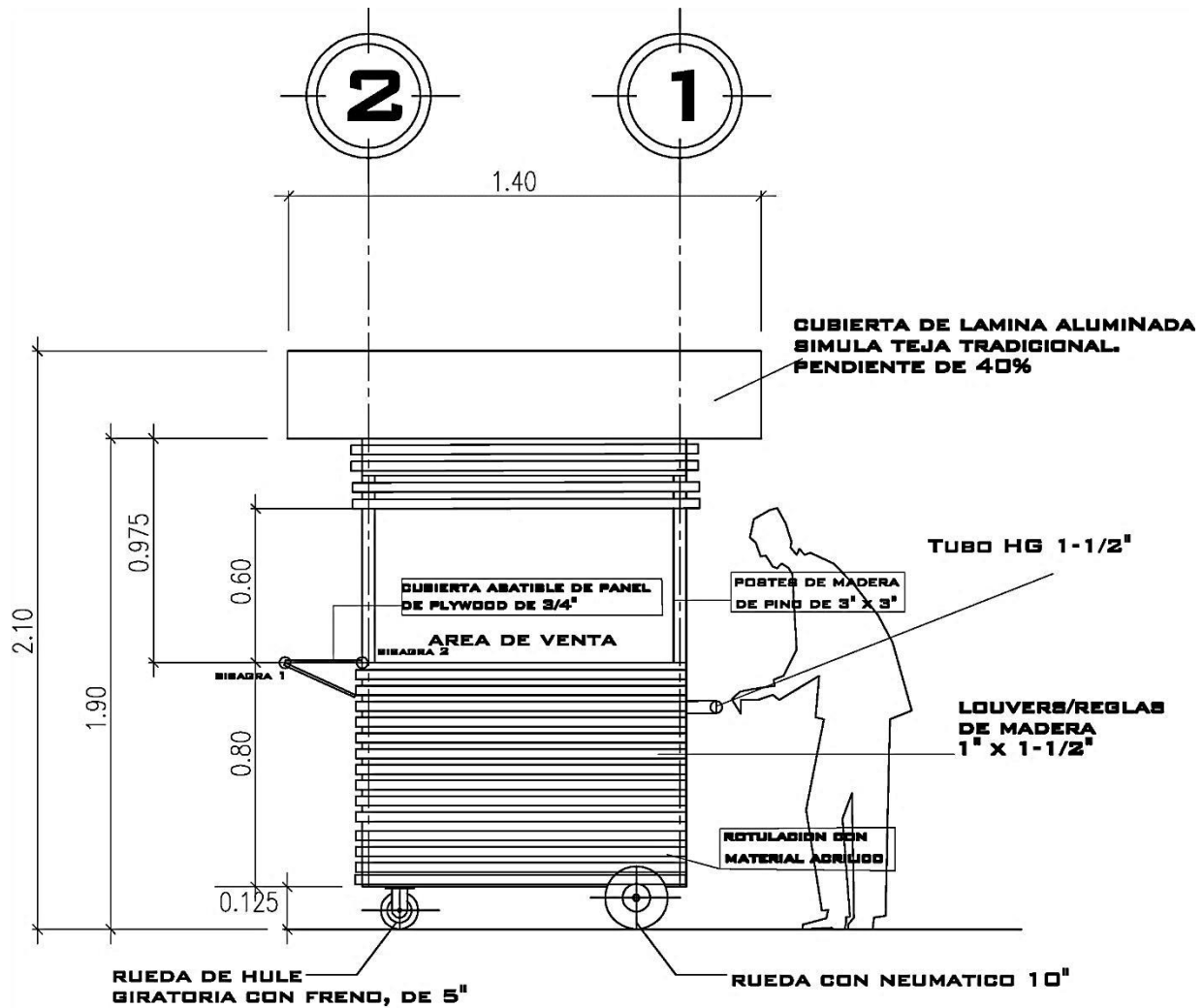
FACHADA CONSTRUCTIVA COTAS EN METROS ESC 1:25
