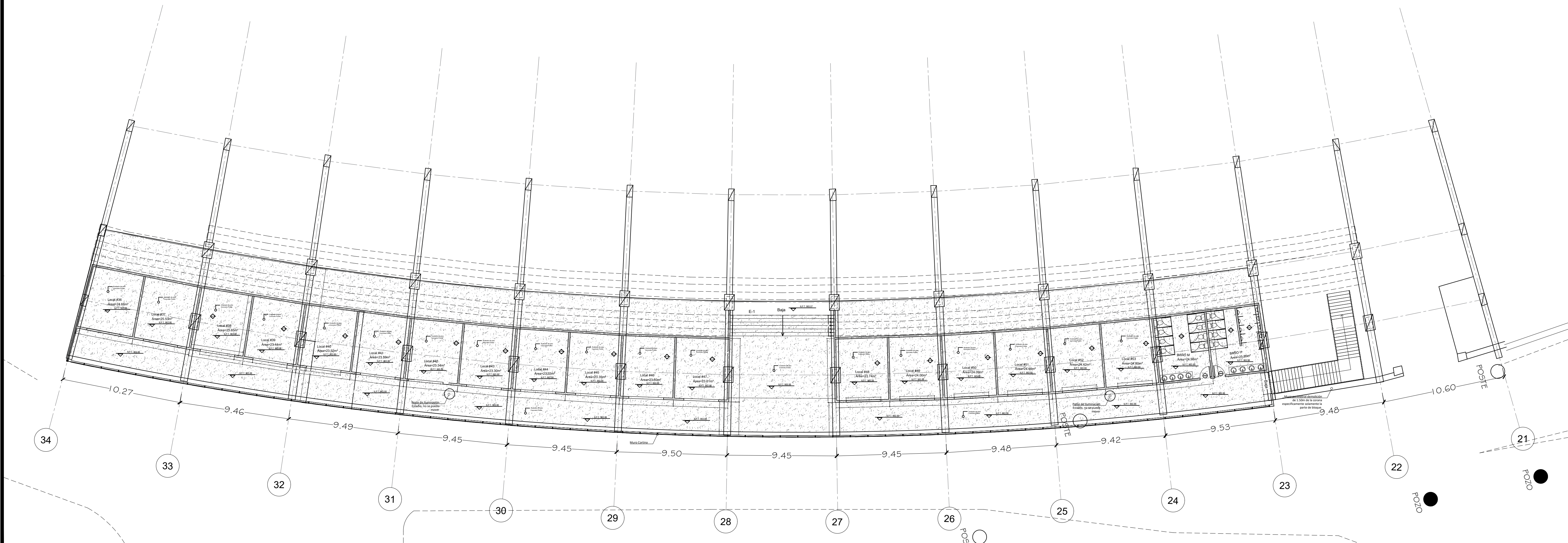
PLANTA ARQUITECTÓNICA NIVEL 2 1:1000
