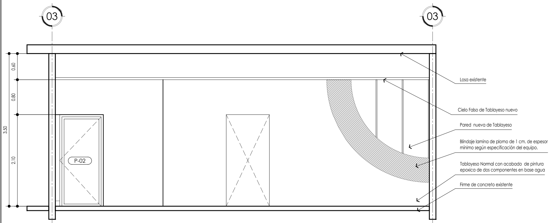
02 SECCIÓN B-B Escala 1:50
