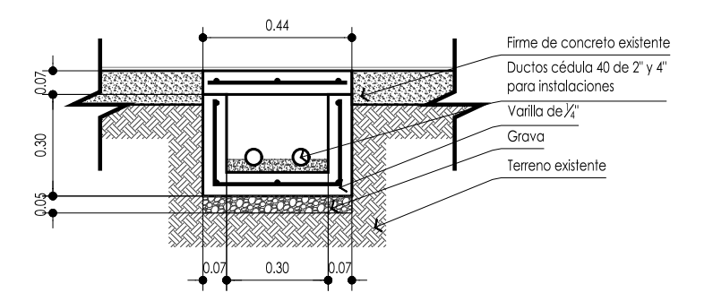
02 D-3 DETALLE DE CANAL DE DUCTOS PARA INSTALACIONES DE MÁQUINA INNOVA PLUS Escala 1:20
