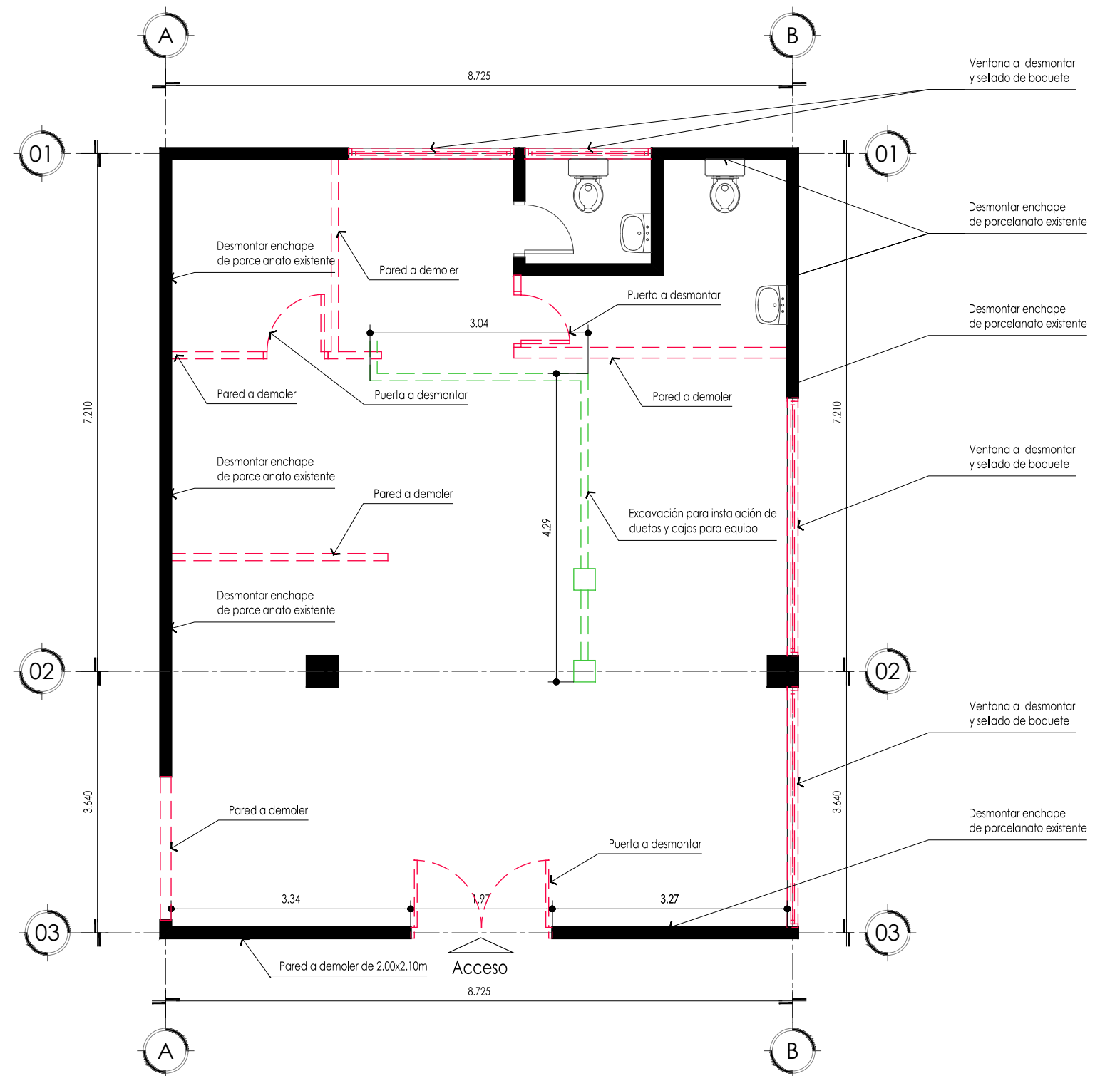
02 PLANTA DE DEMOLICIÓN Escala 1:75
