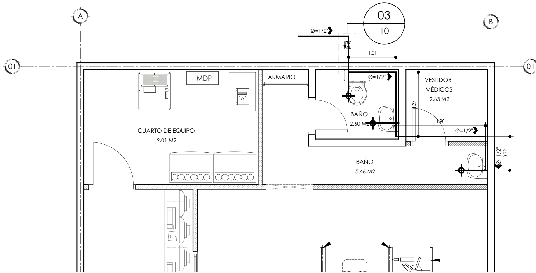
01 PLANTA DE INSTALACIONES DE AGUA POTABLE Escala 1:50
