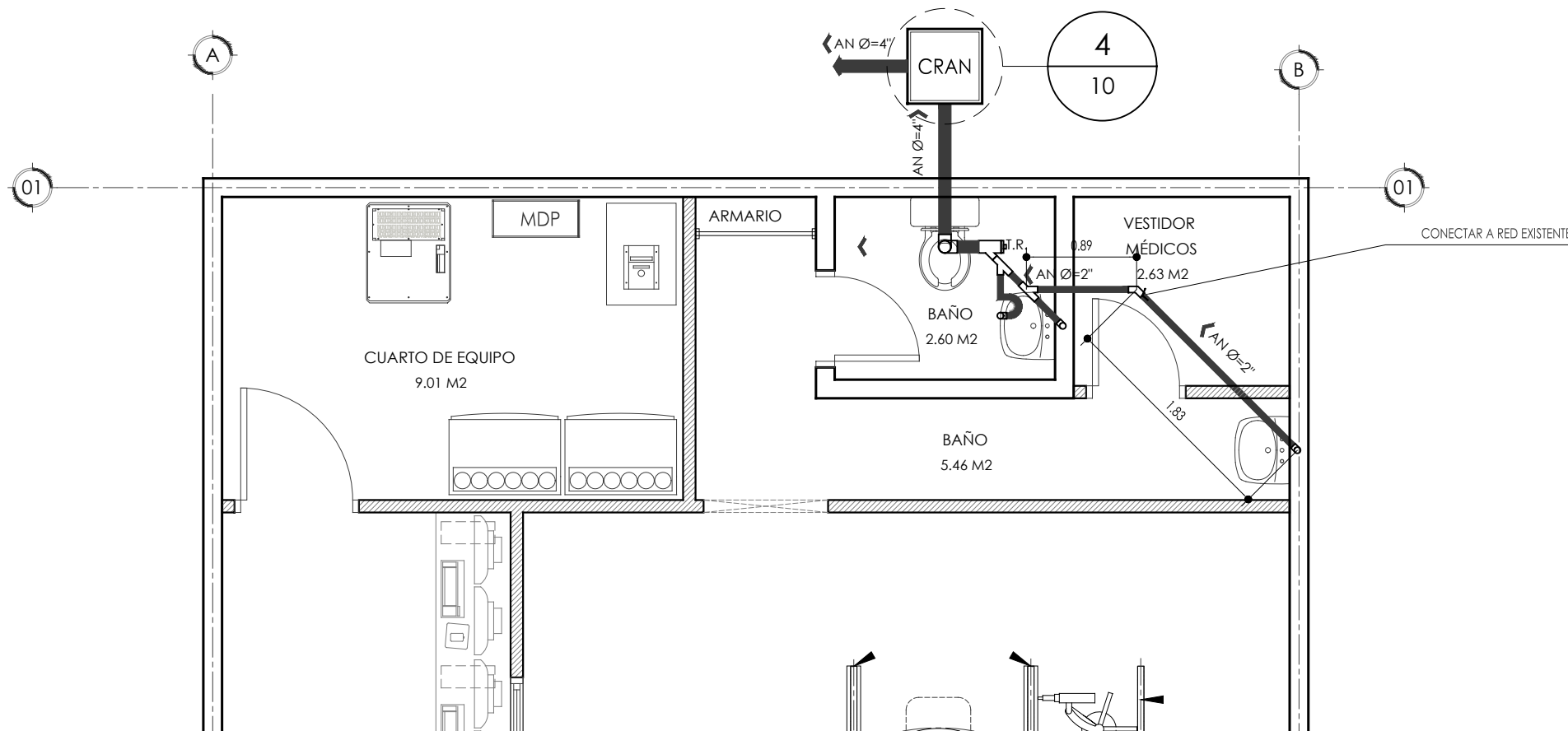
01 PLANTA DE INSTALACIONES DE AGUAS NEGRAS Escala 1:75
