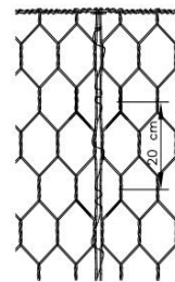
Detalle de la Costura
