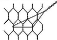
Detalle del Atirantamiento
