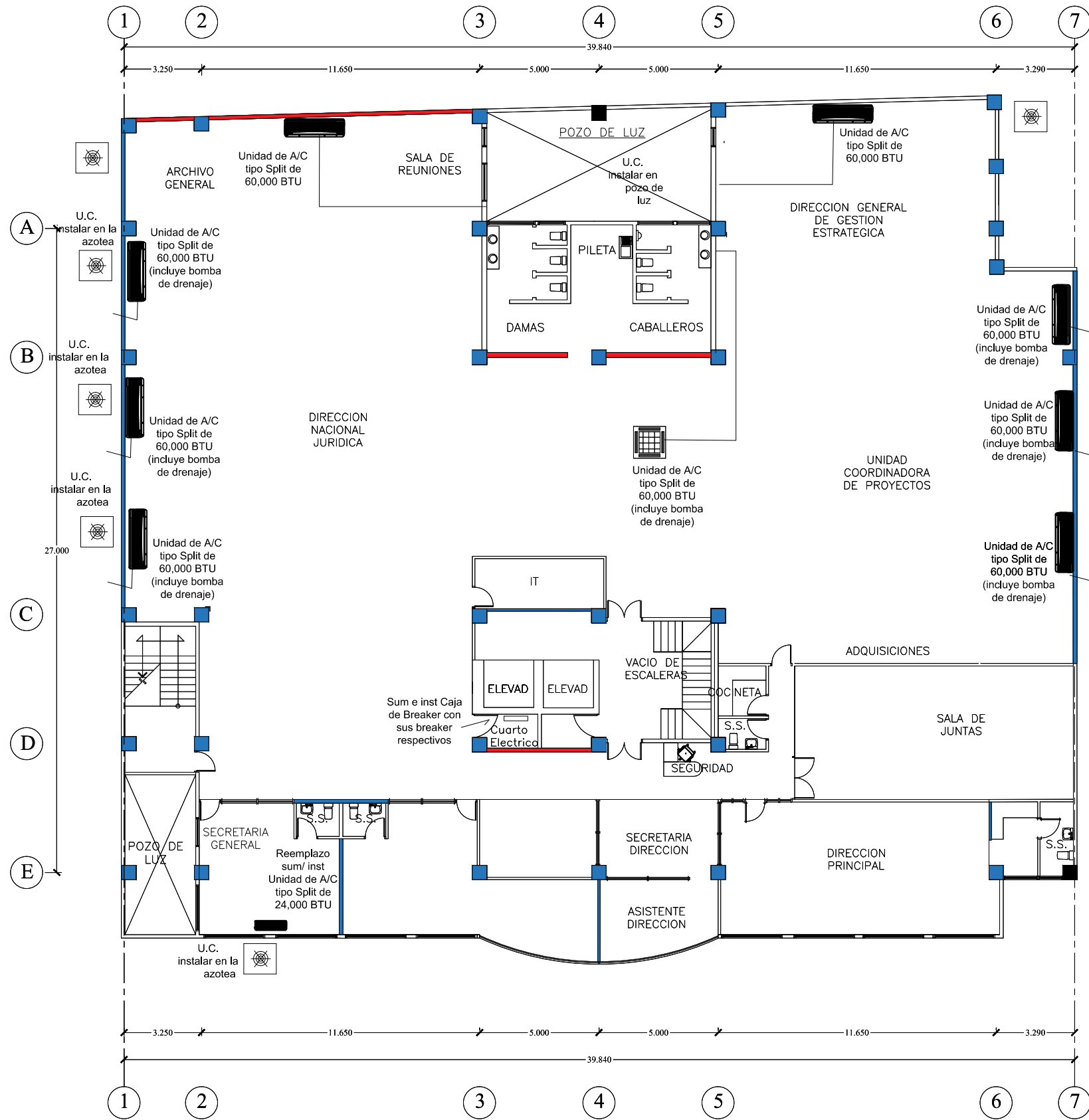
Esquema de Ubicación de tubo de Drenaje PVC ESCALA 1/250 CUARTO NIVEL
