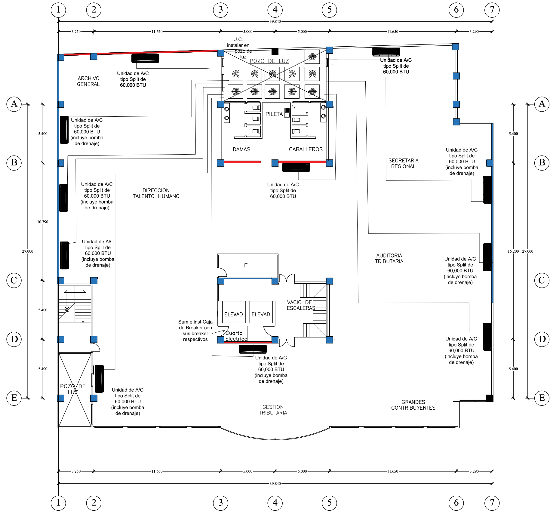
ESQUEMA DE TUBERIA PVC ESCALA 1/250 TERCER NIVEL
