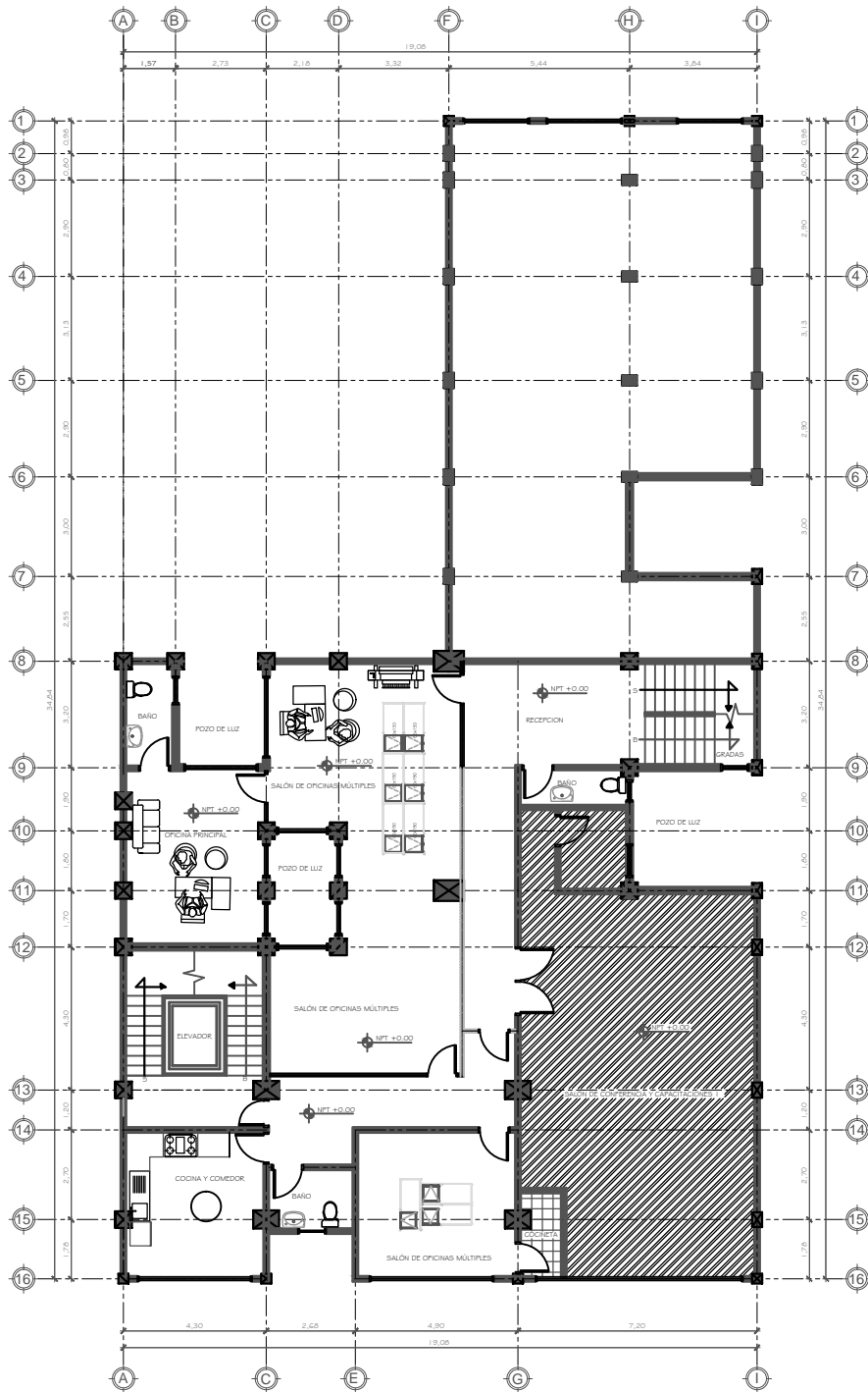
PLANO DE UBICACIÓN DE SALON DE CAPACITACIONES Z 5TO NIVEL ESC 1/100
