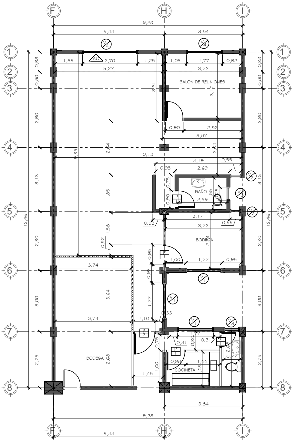
PLANTA CONSTRUCTIVA DE SITUACIÓN ACTUAL DE SALÓN DE CAPACITACIONES
