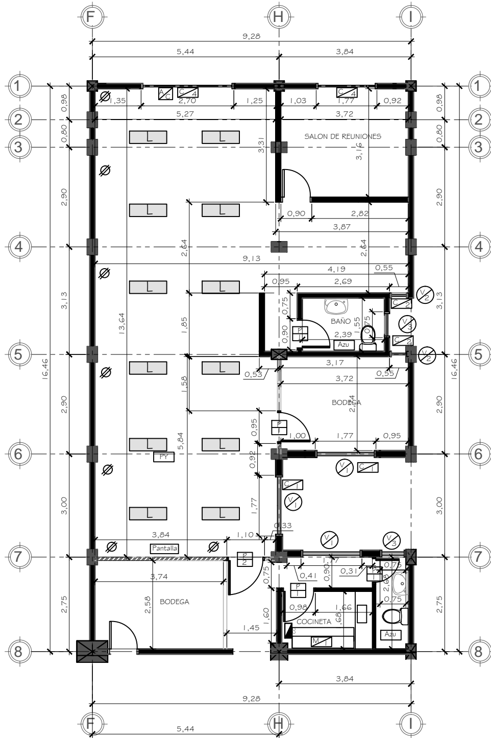
PLANTA CONSTRUCTIVA DE REMODELACIÓN DE SALON DE CAPACITACIONES
