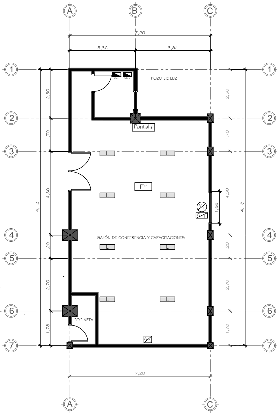
PLANTA CONSTRUCTIVA DE REMODELACIÓN DE SALON DE CAPACITACIONES NIVEL 5
